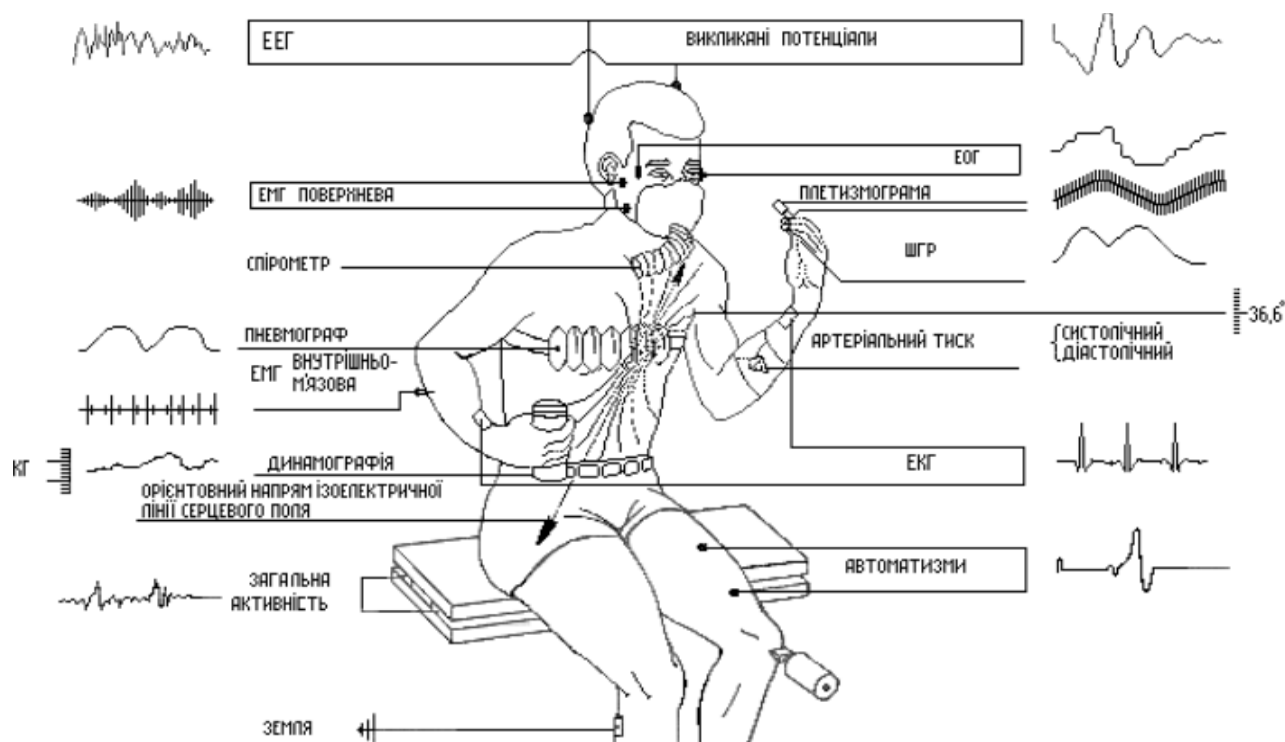
Рис. 2.1.3. Багатоканальна контрольно-вимірювальна система найпоширеніших фізіологічних параметрів індивіда
